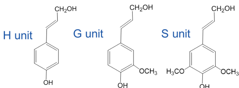
Figure 1.2. Structural units in lignin (Sjöström, 1981).
