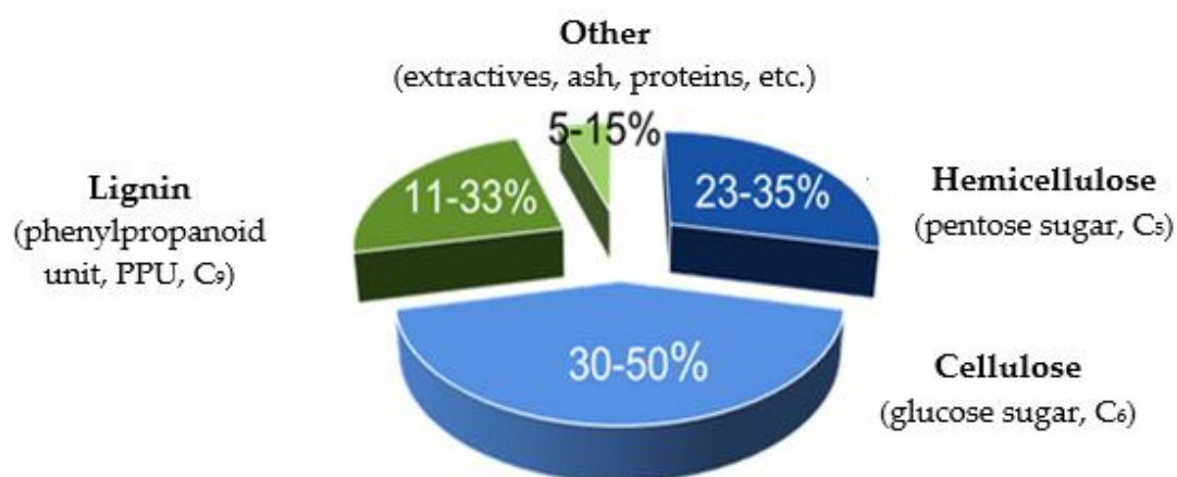
Figure 1.1. Typical composition of the lignocellulosic biomass (Sjöström and Alén, 1998).
